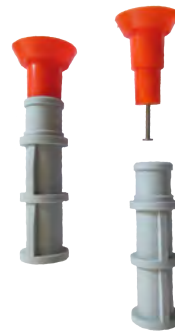
Betonhülse inkl. Sichtnagelstopfen
