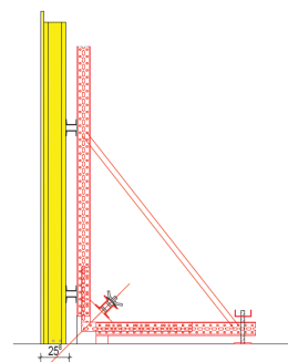
Bockabstand 1.25 m
