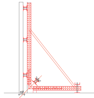
Bockabstand 1.35 m
