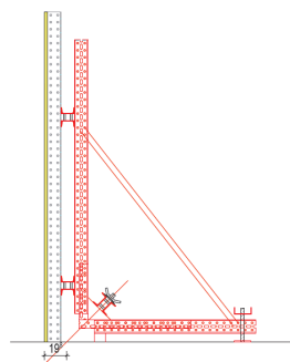
Bockabstand 1.25 m
