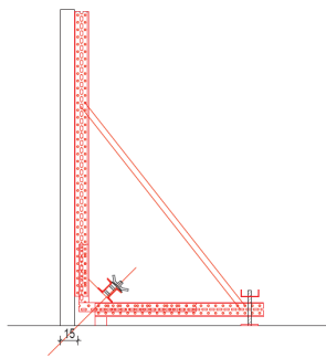
Bockabstand 1.0 m
